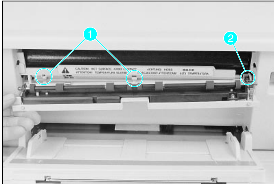
Fuser Door
